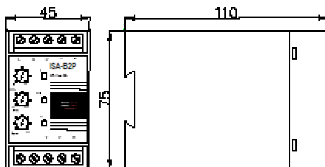
9-1 Gehäuse S1
