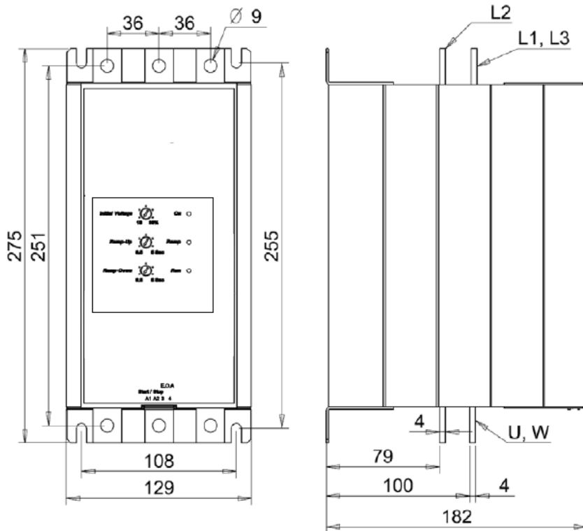
9-5 Gehäuse S5
