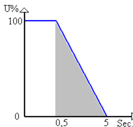
6-3 Stopprampenzeit
