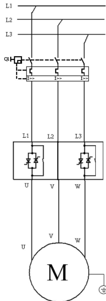
5-3 Anschlussdiagramm für den Hauptstromkreis
