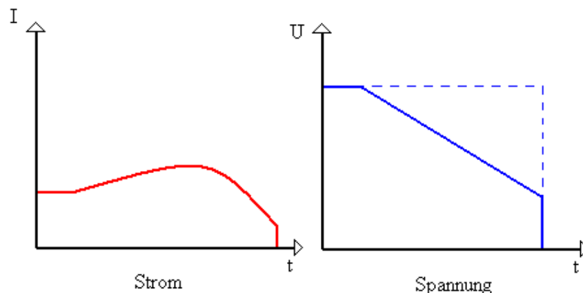
3-2 Sanft-Stopp Charakteristika
